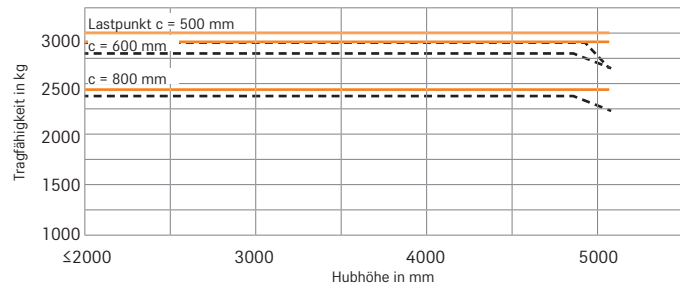
RX 60-30 Teleskop/NiHo-Hubgerüst
