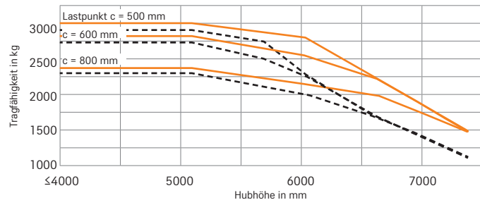
RX 60-30 Dreifach-Hubgerüst
