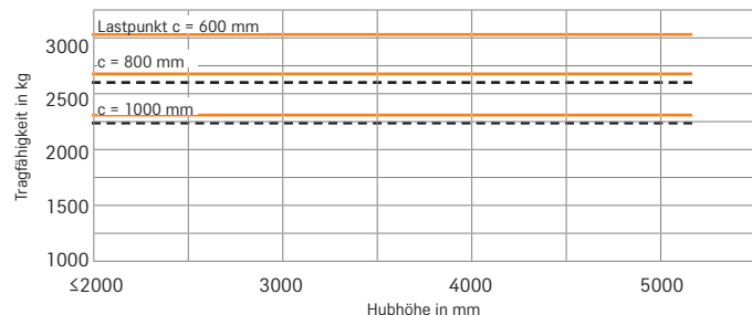
RX 60-30L/600 Teleskop/NiHo-Hubgerüst
