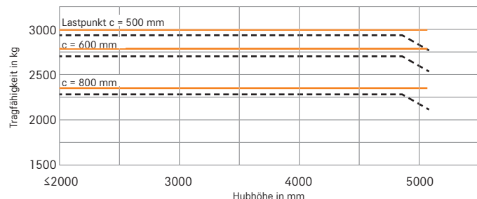
RX 60-30L Teleskop/NiHo-Hubgerüst
