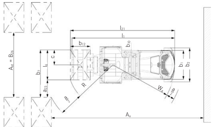
MX-X mit Teleskoptisch und induktiver Führung - Draufsicht
