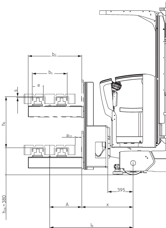
MX-X mit hohem Teleskoptisch - Seitenansicht
