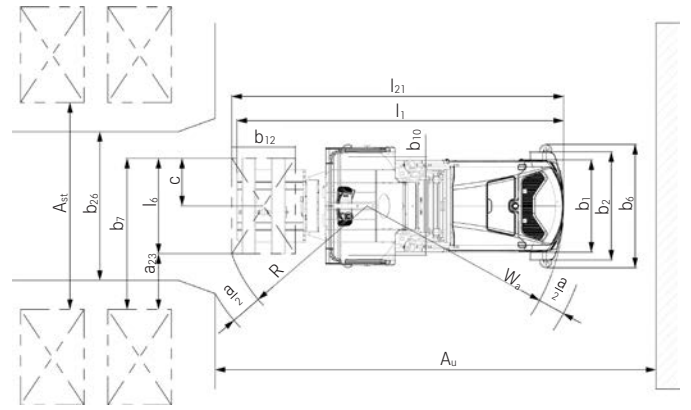
MX-X mit Teleskoptisch und mechanischer Führung - Draufsicht
